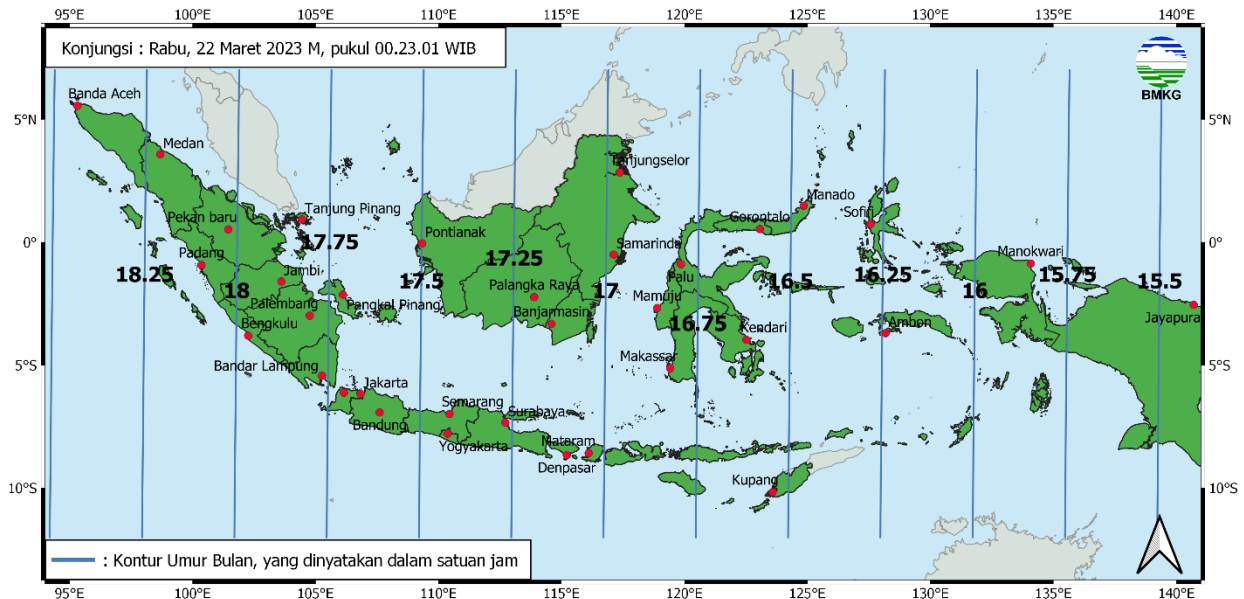
Gambar 6. Peta umur bulan tanggal 22 Maret 2023 untuk pengamat di Indonesia
