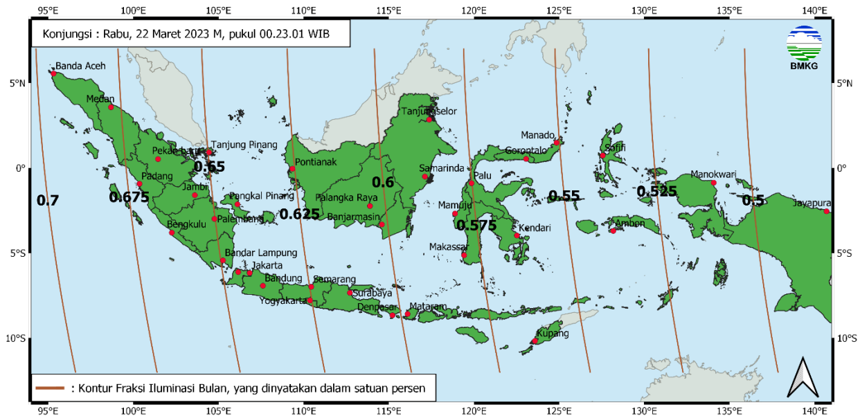
Gambar 10. Peta fraksi illuminasi bulan tanggal 22 Maret 2023 untuk pengamat di Indonesia
