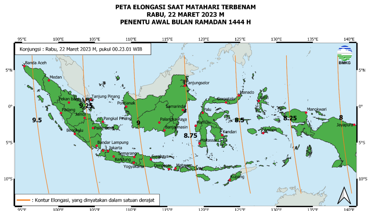
Gambar 4. Peta elongasi tanggal 22 Maret 2023 untuk pengamat di Indonesia
