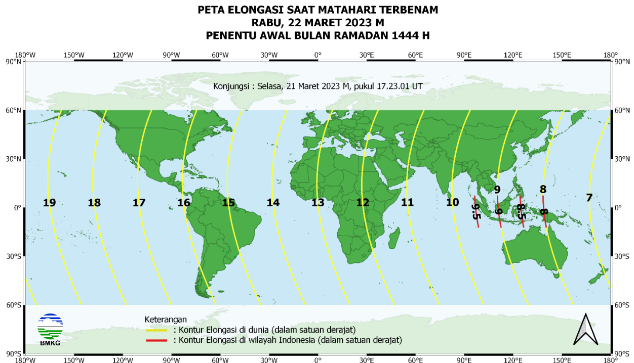
Gambar 3. Peta elongasi tanggal 22 Maret 2023 untuk pengamat antara 60° LU sampai dengan 60° LS
