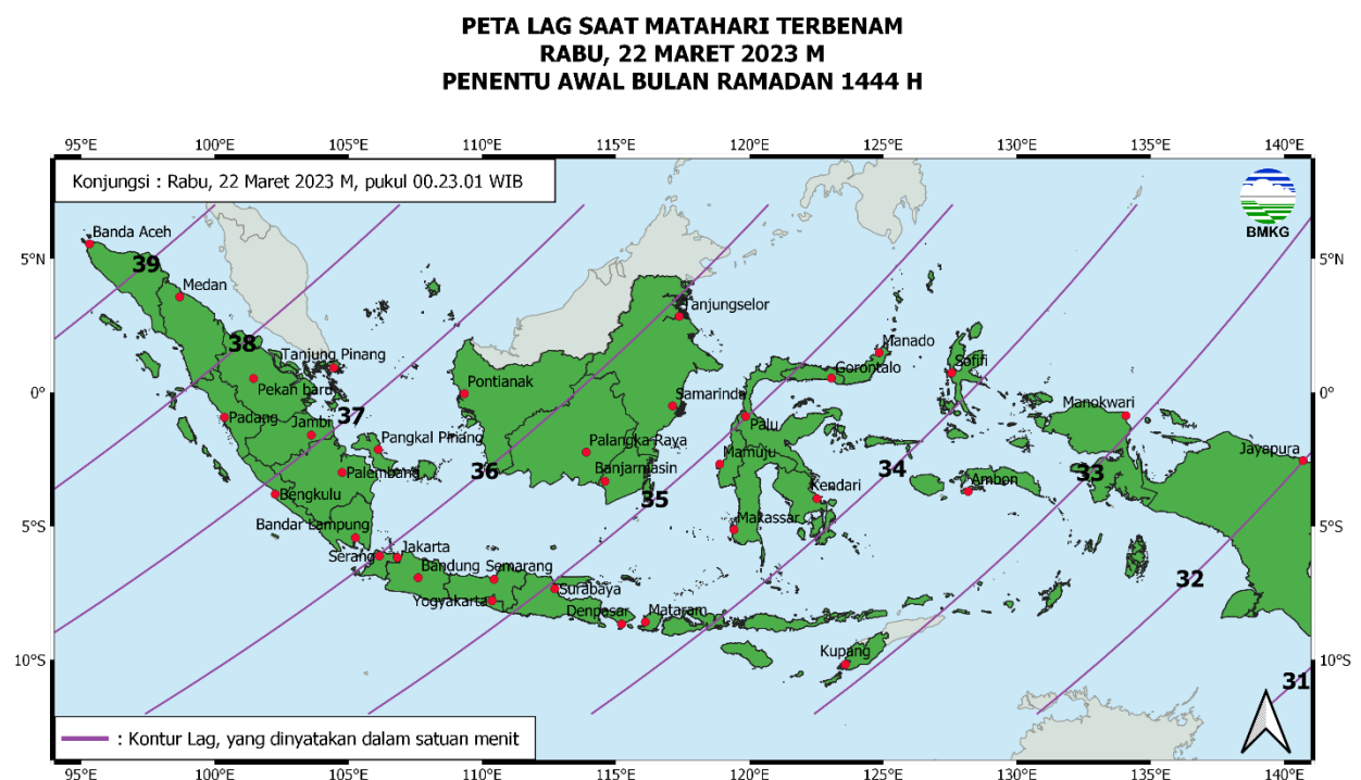
Gambar 8. Peta lag tanggal 22 Maret 2023 untuk pengamat di Indonesia
