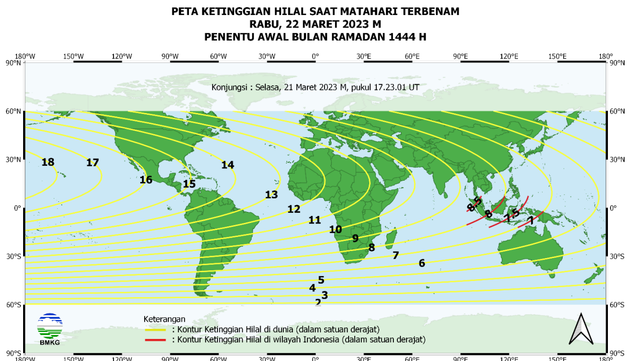
Gambar 1. Peta ketinggian Hilal tanggal 22 Maret 2023 untuk pengamat antara 60^\circ LU sampai dengan 60^\circ LS
