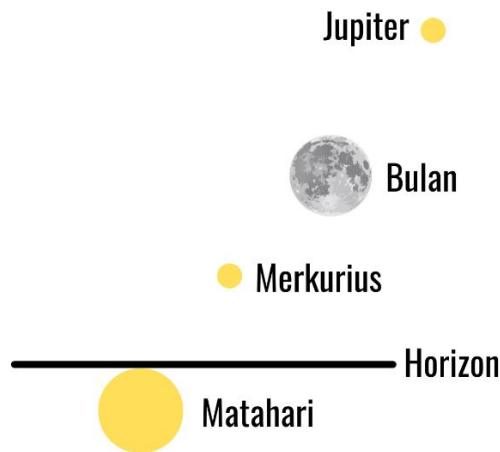
Gambar 11. Ilustrasi posisi Bulan, Merkurius, dan Jupiter saat Matahari terbenam
