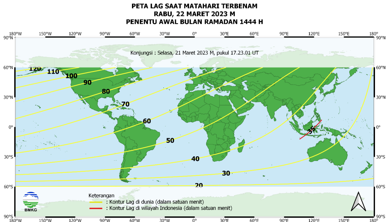
Gambar 7. Peta lag tanggal 22 Maret 2023 untuk pengamat antara 60° LU sampai dengan 60° LS
