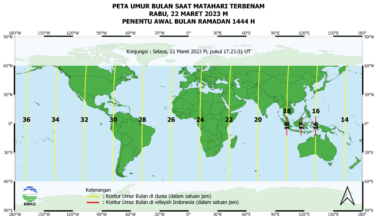
Gambar 5. Peta umur bulan tanggal 22 Maret 2023 untuk pengamat antara 60° LU sampai dengan 60° LS
