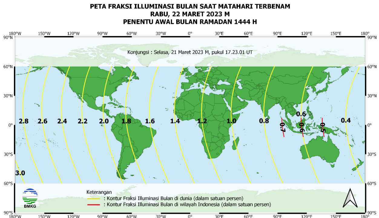
Gambar 9. Peta fraksi illuminasi bulan tanggal 22 Maret 2023 untuk pengamat antara 60° LU s.d. 60° LS
