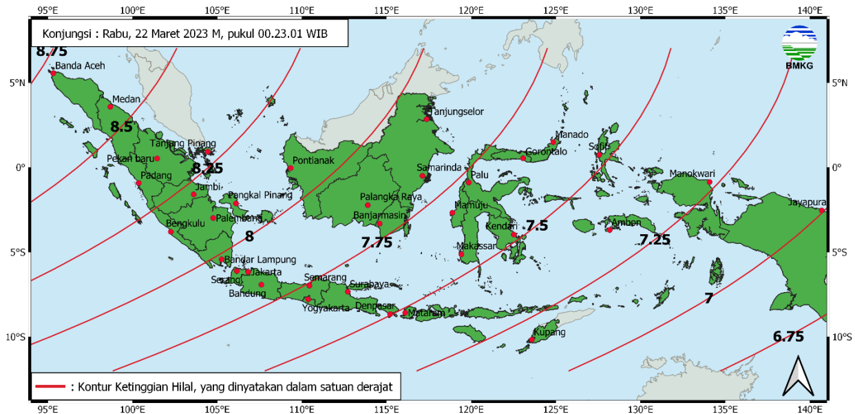
Gambar 2. Peta ketinggian Hilal tanggal 22 Maret 2023 untuk pengamat di Indonesia
